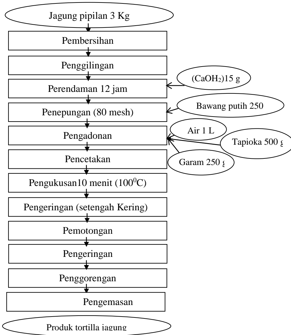
Gambar 4. Diagram alir Pembuatan Tortilla Jagung KWT Kemuning II Sumber: Usaha KWT Kemuning II
