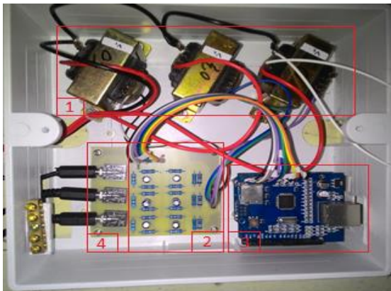
Gambar 2 IoT pembaca besaran listrik tiga fasa
