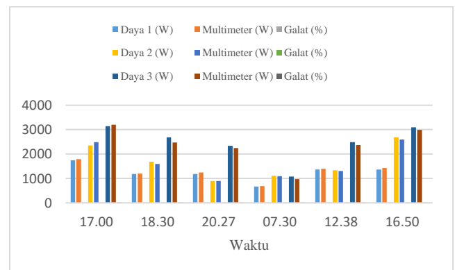
Gambar 3 Hasil pengujian daya pada IoT
