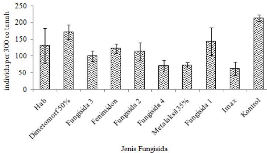
Gambar 1. Kelimpahan (nilai tengah \pm SE) seluruh nematoda pada tanaman jagung yang mendapat perlakuan benih dengan berbagai jenis fungisida.
