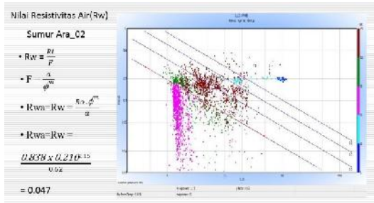
Gambar 6. Nilai Resistivitas air pada sumur Ara_02 menggunakan metode Picket plot.
