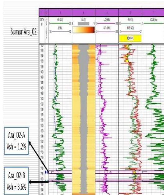
Gambar 4. Zona Ara-02-A dan Ara-02-B sebagai zona potensial sumur Ara-02.
