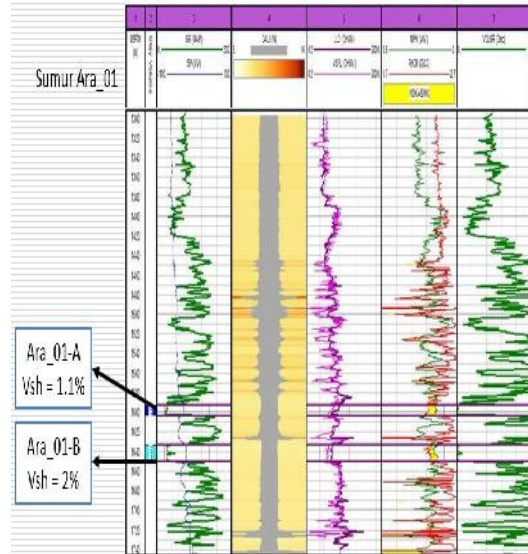
Gambar 3. Zona Ara-01-A dan Ara-01-B sebagai zona potensial sumur Ara-01.
