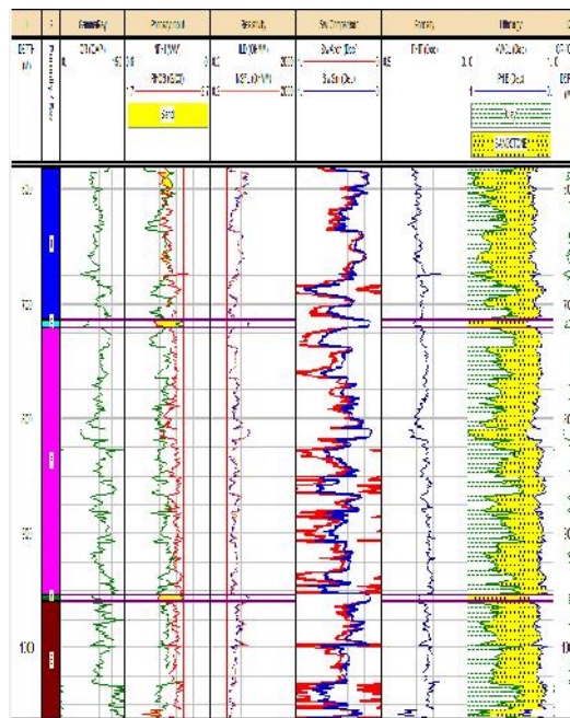
Gambar 4. Hasil Analisa Porositas dan Sw T-RX1
