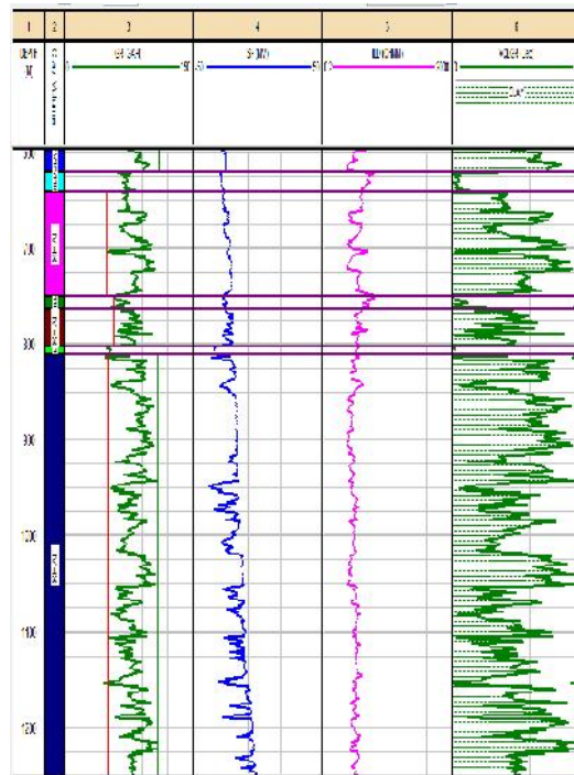
Gambar 3. Hasil Interpretasi Kuantitatif Volume Shale pada sumur T-RX3
