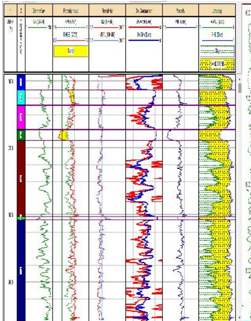
Gambar 5. Hasil Analisa Porositas dan Sw T-RX2
