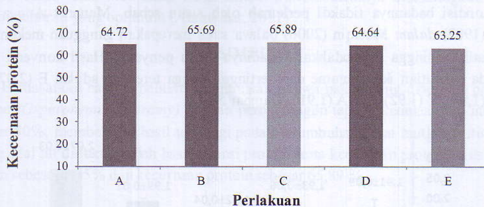
Gambar 3. Kecernaan protein
