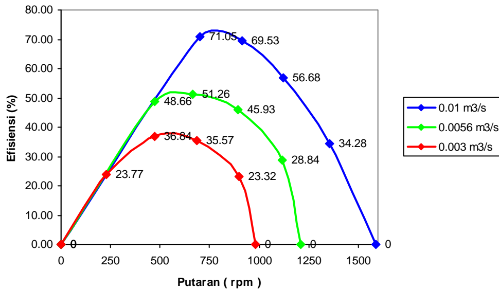
Gambar 12. Grafik hubungan antara efisiensi terhadap putaran turbin untuk berat roda gila 1,2 kg.
