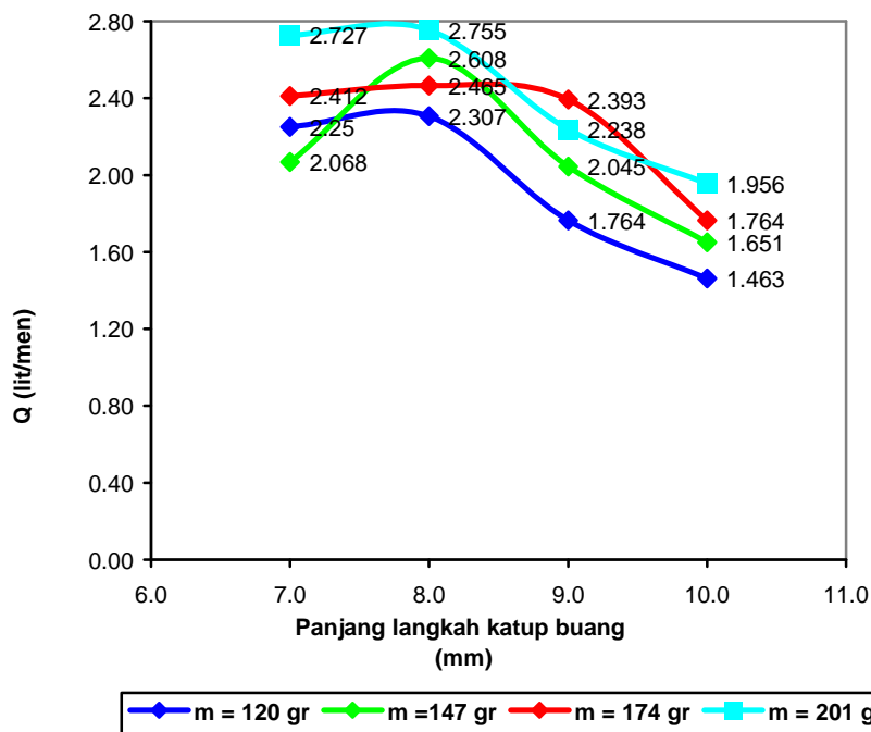
Gambar 5. Grafik hubungan antara laju aliran volume air yang disalurkan terhadap panjang langkah katup buang untuk tinggi head pemompan 7 m
