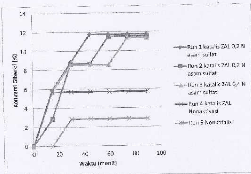
Gambar 2. Hubungan waktu vs konversi Gliserol pada ketiga variasi aktivasi ZAL. Rasio Gliserol dan Asam Asetat 1 mol : 7 mol, temperatur 100 ° C, tekanan 1 atm, dengan jumlah katalis adalah 3 % berat asam asetat.
