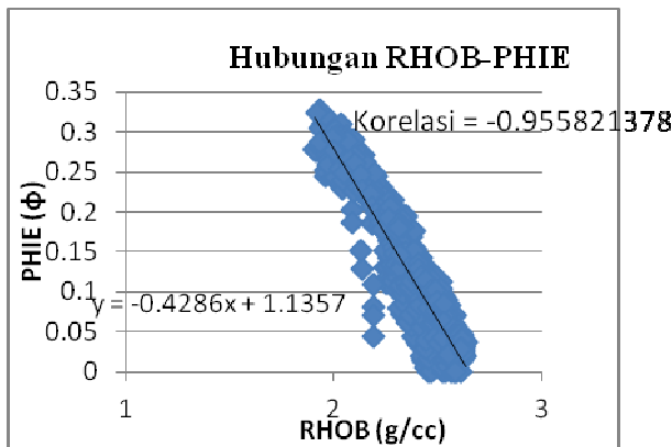
Gambar 20. Hubungan RHOB-PHIE
