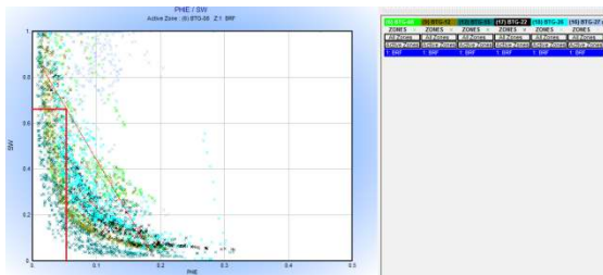
Gambar 19. Penentuan Cutoff Saturasi Air ( S_w )
