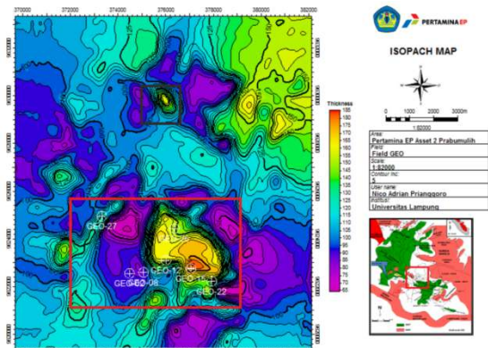
Gambar 9. Peta Isopach Lapangan GEO
