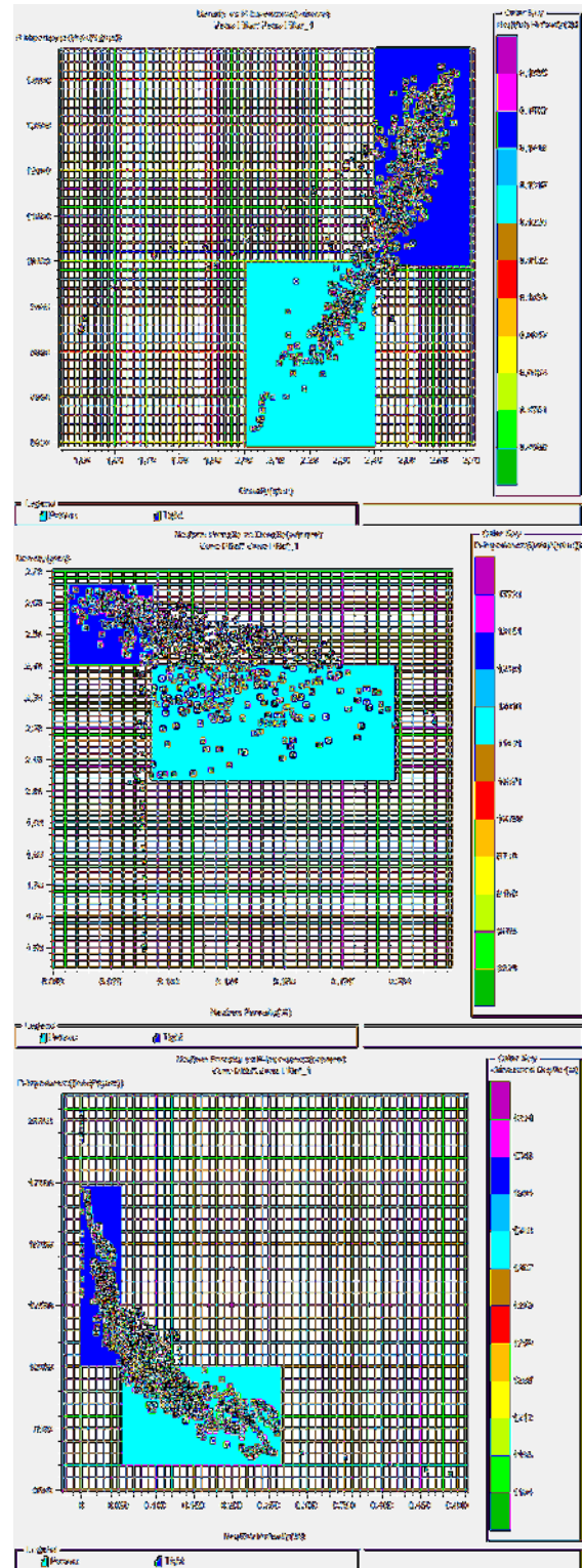
Gambar 5. Analisis crossplot Den-Pimp, Den-Neu dan Pimp-Neu
