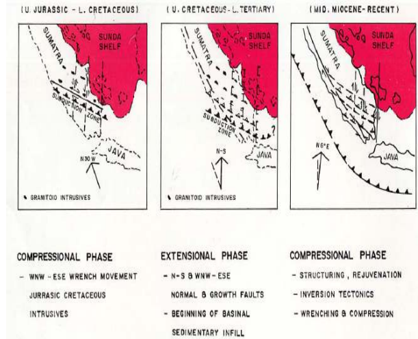
Gambar 2. Fase Tektonik Cekungan Sumatera Selatan (Pulunggono, dkk., 1992)
