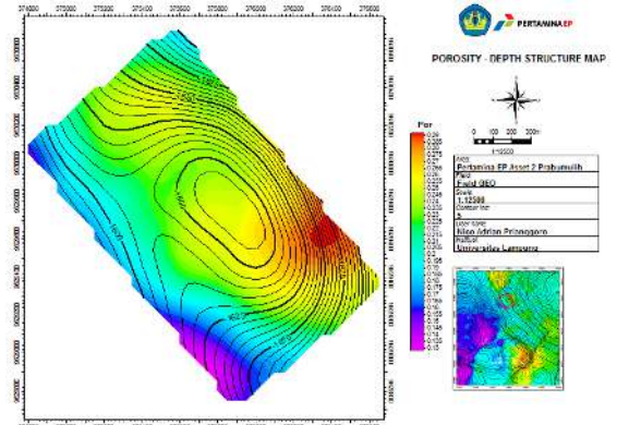
Gambar 21. Peta Sebaran Porositas Lapangan GEO dan Fokus Area Outstep
