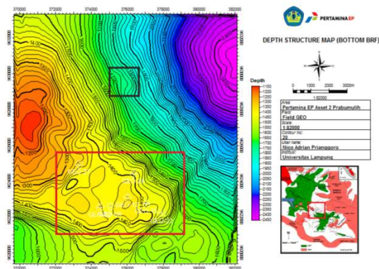
Gambar 8. Peta struktur kedalaman Bottom BRF Lapangan GEO
