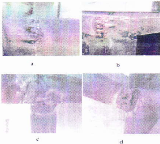
Gambar 4. Hasil pengelasan
