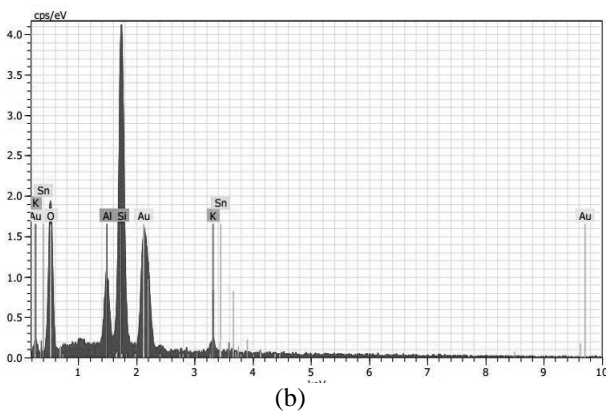
Gambar 3. Spektrum EDX dari (a) Silika Berpori ; (b) Fotokatalis SnO 2 -SiO 2 0,025
