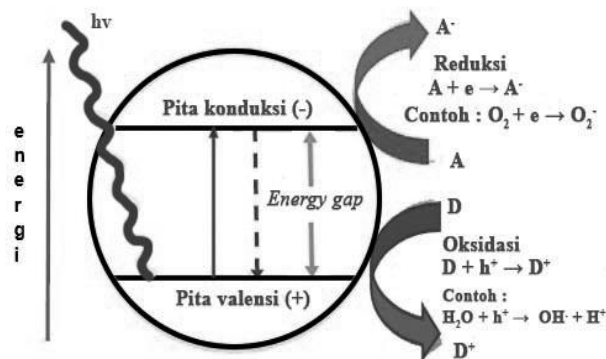
Gambar 5. Mekanisme Fotokatalis [28]
