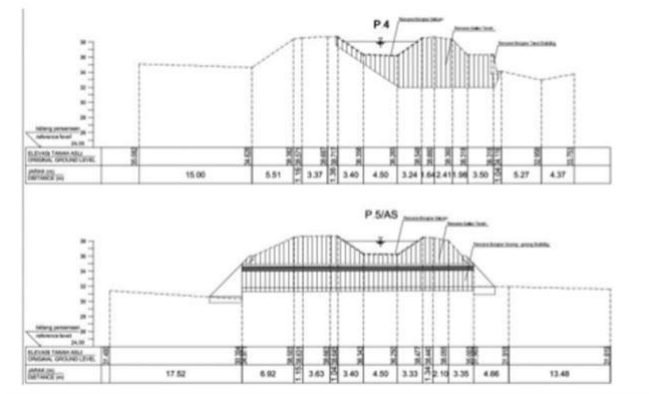
Gambar 4.3. Pemetaan Situasi Saluran Primer Raman Utara
