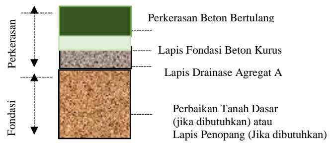
• Gambar 1. Tipikal Struktur Perkerasan Kaku Terpilih
