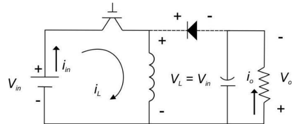
Gambar 6. Topologi Konverter Buck Boost saklar on
