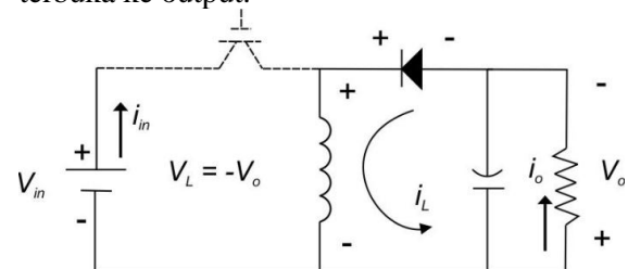
Gambar 7. Topologi Konverter Buck Boost saklar off
