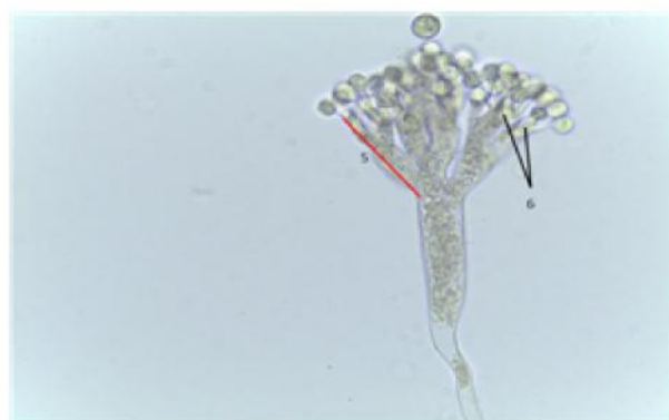
Gambar 1. Pengamatan Morfologi Konidia dan Konidiofor. (1) Tebal konidia, (2) Panjang konidia, (3) Dinding sel, (4) Panjang konidiofor, (5) Panjang tangkai konidiofor, (6) Jumlah percabangan.
