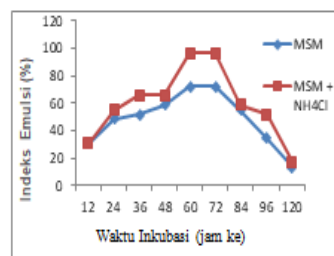
Gambar 4. Waktu Optimum Produksi Biosurfaktan dengan Indeks Emulsifikasi (IE 24 )
