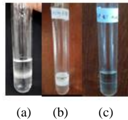
Gambar 1. Indeks Emulsifikasi ( IE_{24} ) Isolat ALP E1 pada (a) n-heksana (b) Benzena (c) Aquades
