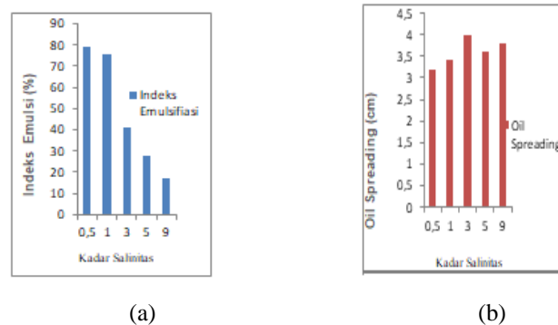
Gambar 6. (a) Indeks Emulsifikasi ( IE_{24} ) pada Optimasi Produksi Kadar Salinitas Biosurfaktan (b) Uji Oil Spreading pada Optimasi Produksi Kadar Salinitas Biosurfaktan
