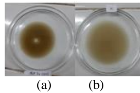
Gambar 3. Uji Oil Spreading Isolat Indigen ALP E1 pada (a) Kontrol (b) Sampel
