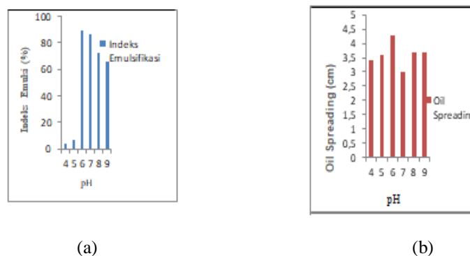
Gambar 5. (a) Indeks Emulsifikasi (IE 24 ) pada Optimasi Produksi pH Biosurfaktan (b) Uji Oil Spreading pada Optimasi Produksi pH Biosurfaktan
