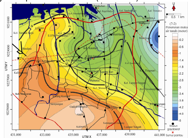
Gambar 10. Penurunan muka air sumur bor daerah Semarang 2002 - 2005
