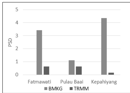
Gambar 4 Perbandingan puncak frekuensi antar stasiun FFT
