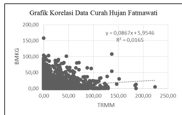
Gambar 3 Contoh hasil analisis korelasi BMKG dan TRMM stasiun Fatmawati
