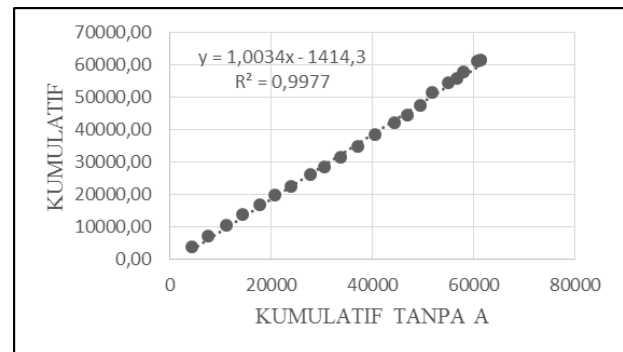
Gambar 2 Hasil uji konsistensi stasiun Fatmawati
