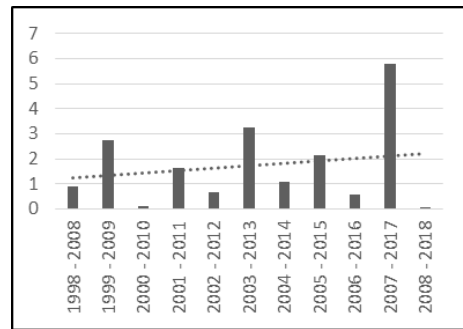
Gambar 7 Grafik pertumbuhan pengaruh anomali iklim Kepahiyang BMKG
