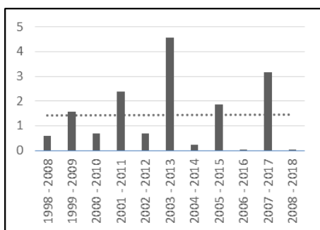
Gambar 6 Grafik pertumbuhan pengaruh anomali iklim Fatmawati BMKG
