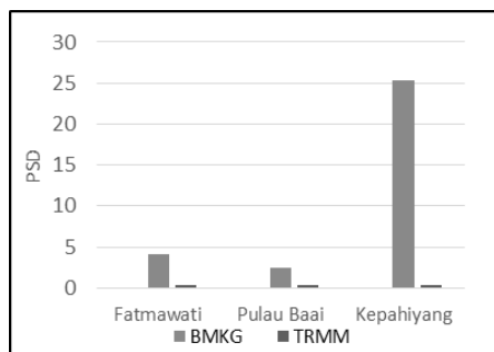
Gambar 5 Perbandingan puncak frekuensi antar stasiun Lomb
