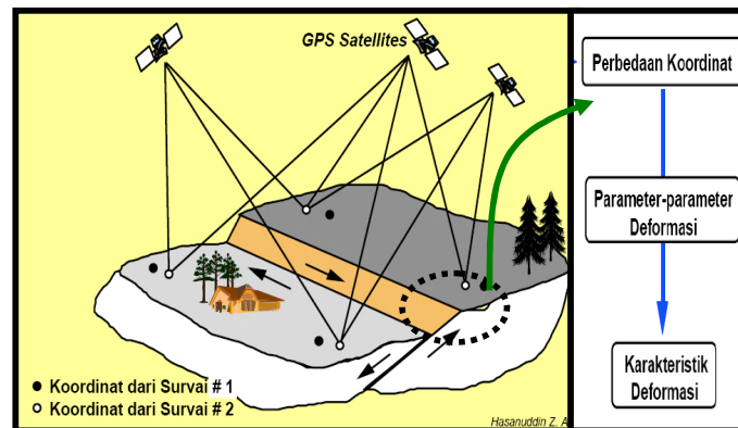
Gambar 4. Studi Deformasi Pada Daerah Sesar
