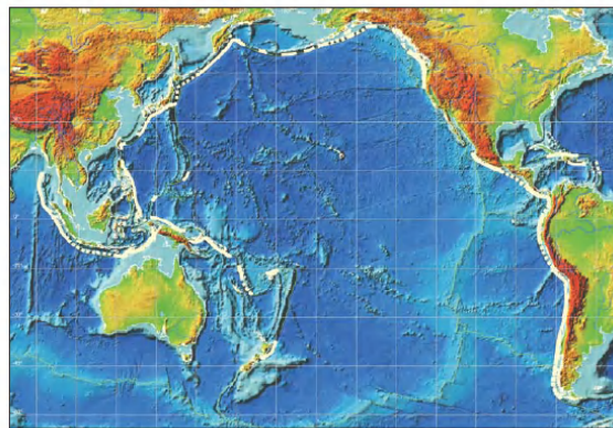
Gambar 2. Garis putih merupakan jalur tumbukan ketiga lempeng besar dunia
