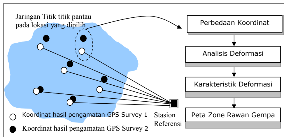
Gambar 7. Prinsip Penentuan Gerakan Tanah Dengan Metode Survei GPS
