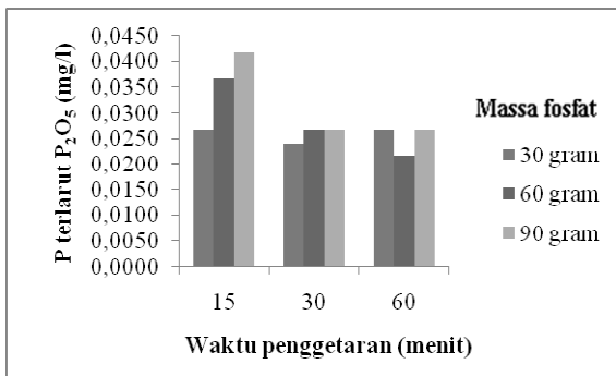
Grafik 1. Hubungan massa fosfat dan waktu penggetaran terhadap kadar P terlarut sampel cair
