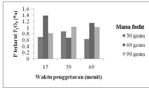
Grafik 2. Hubungan massa fosfat dan waktu penggetaran terhadap kadar P terlarut sampel padat
