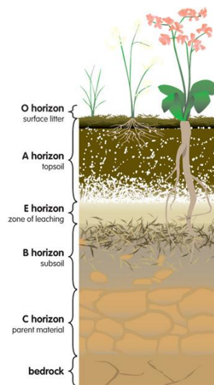
Gambar 14. Profil Tanah
