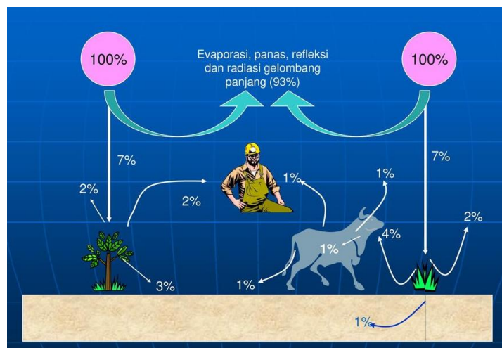
Gambar 3. Penyebaran Energi
