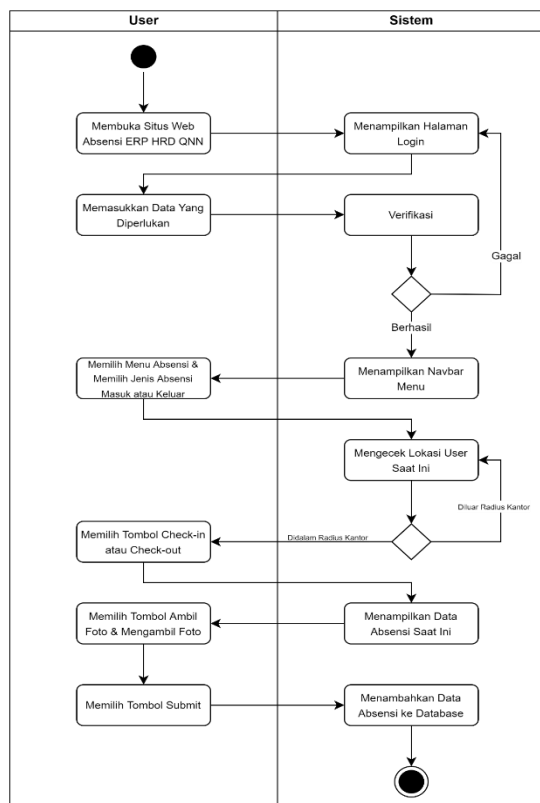
Gbr.3 Activity Diagram Melakukan Absensi
