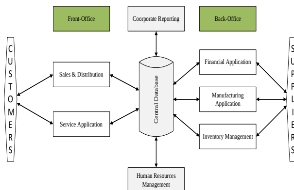
Gbr.1 Arsitektur ERP Secara Umum
