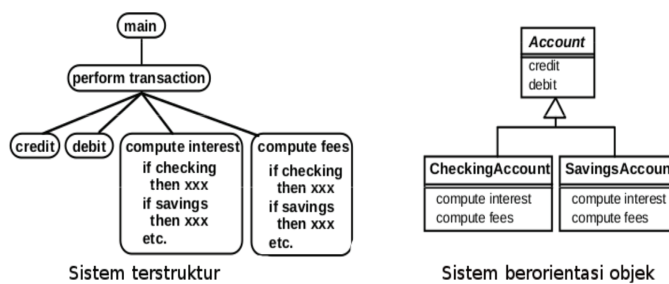
Gambar 1. Perbedaan sistem terstruktur dan sistem berorientasi objek.
