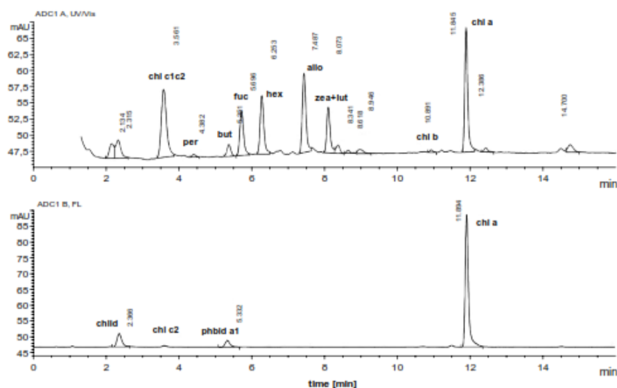
Gambar 1. Kromatogram dari pigmen klorofil dan karotenoid dengan menggunakan UV/Vis detector ( gambar atas ), dan degradasi produk klorofil dengan menggunakan spectrofluorimetric detector ( gambar bawah ). Dari nilai puncak tunggal kita dapat menentukan kualitas (posisi puncak) dan kuantitas (area puncak) dari pigmen fitoplankton (Gitelson et al. , 2000)
