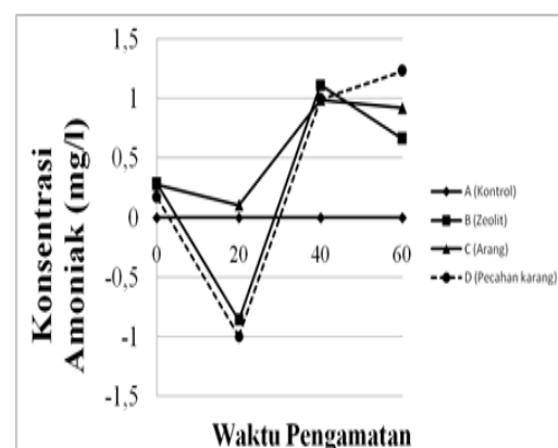
Gambar 2. Konsentrasi amonia (mg/l) penggunaan filter yang berbeda pada sistem resirkulasi.
