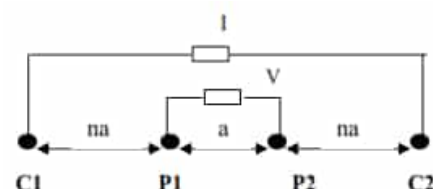
Gambar 1. Konfigurasi Wenner-Schlumberger (Kanata, 2008).
