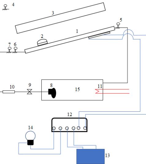
Gambar 3. Skema rangkaian pengujian kolektor PV/T
