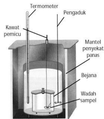
Gambar 3. Skema bomb calorimeter .
