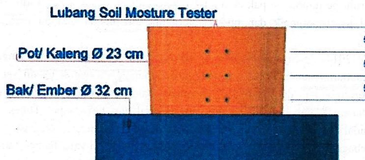
Gambar 2. Sketsa pot tanam tanpa tutup plastik
