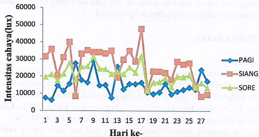
Gambar 6. Intensitas Cahaya di dalam Greenhouse
