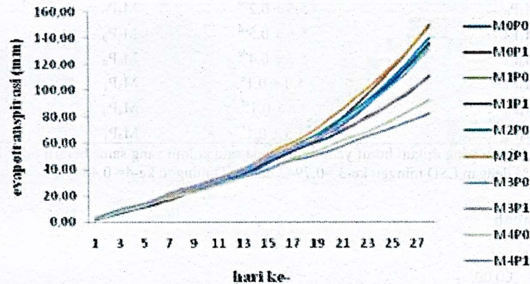
Gambar 7. Evapotranspirasi kumulatif (mm/tanaman) setiap perlakuan
