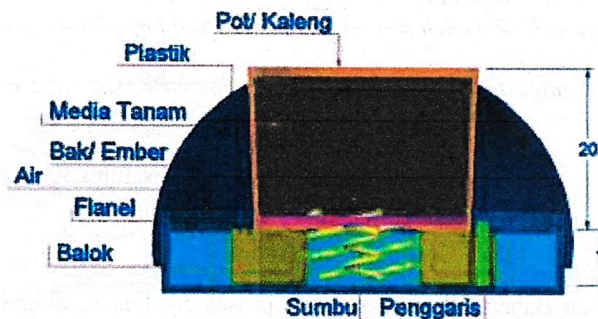
Gambar 1. Sketsa irisan pot tanam
