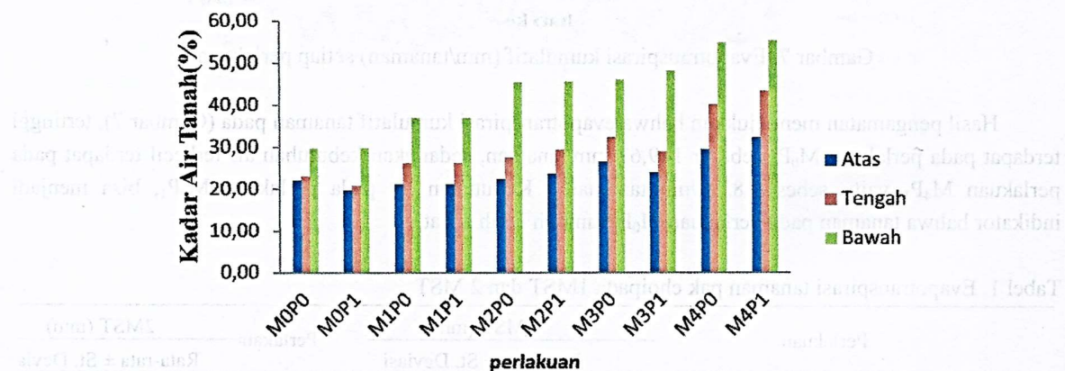
Gambar 8. Kadar air tanah media tanam pada tingkat kedalaman yang berbeda
