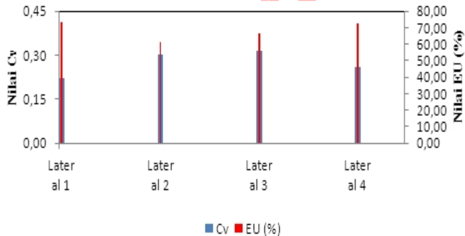
Gambar 5. Hubungan Cv dan EU (%) debit penetes tanpa pompa untuk tiap-tiap lateral
