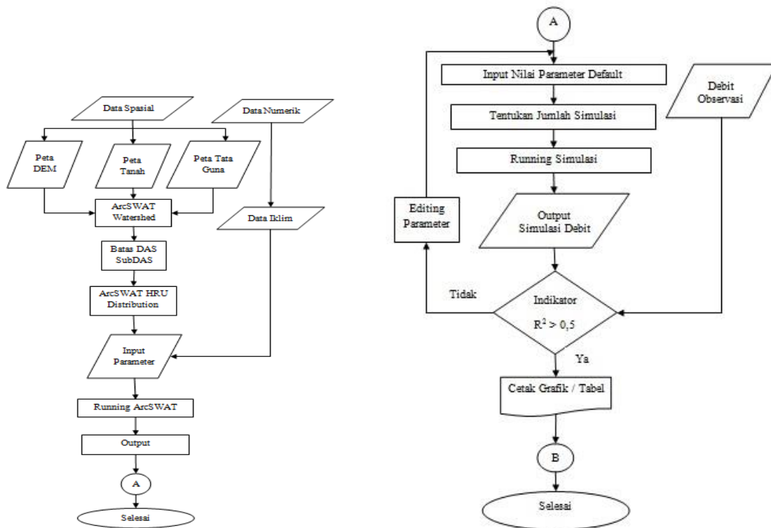
Gambar 1. Diagram Alir Running SWAT dan Kalibrasi Validasi
