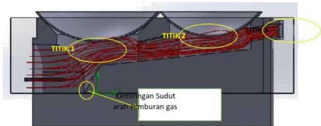
Gambar 3.1 Simulasi Distribusi Temperatur Akibat Kemiringan Sudut Arah Semburan Gas Menggunakan Software SolidWork
