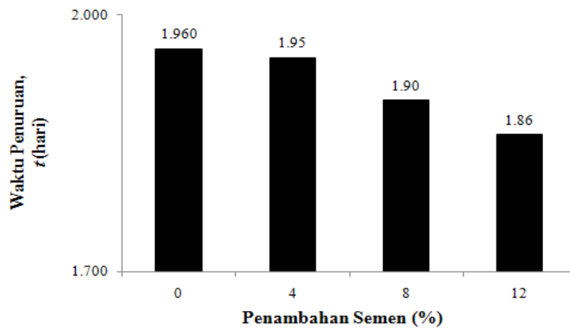
Gambar 7. Grafik pengaruh penambahan semen terhadap waktu penurunan t_{90}
