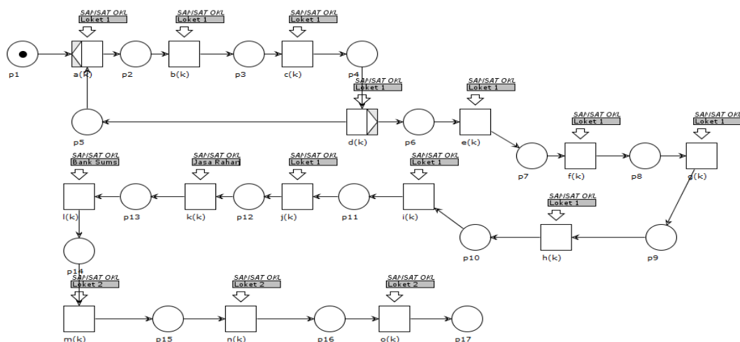
Gambar 1. Alur Petri Net sistem pembayaran pajak kendaraan bermotor jenis 5 tahun di SANSAT Oku Timur 1
