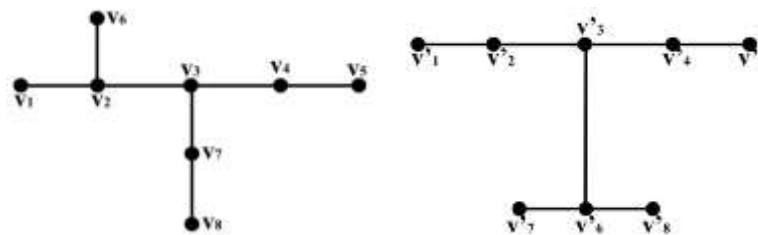
Gambar 3. Graf 3-etil-2-metil Pentana dengan 3-isopropil Pentana yang saling isomorfik
