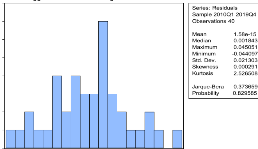
Gambar 4. Uji Normalitas
