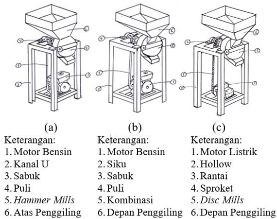
2 Gambar 1. Varian desain konsep, (a) Varian 1, (b) Varian 2, dan (c) Varian 3.
