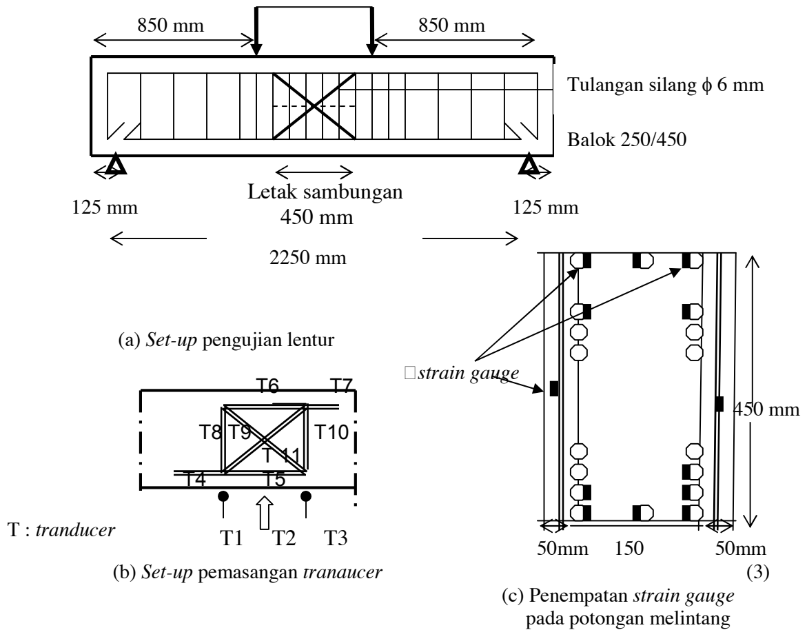
Gambar 2. Set-up pengujian lentur, pemasangan tranducer dan penempatan strain gauge
