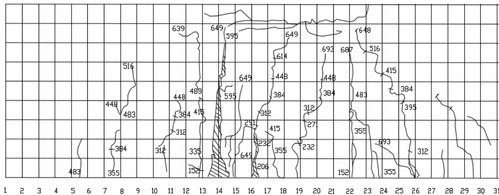
Gambar 9. Pola retak tampak samping
