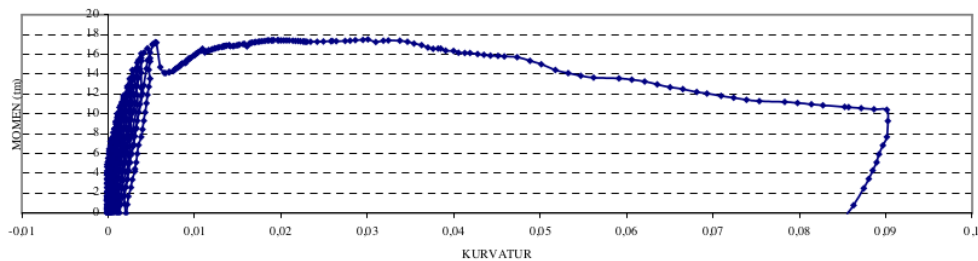
Gambar 6. Lup histerisis momen - kurvatur
