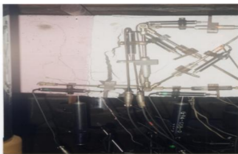
Gambar 7. Penempatan transducer dan gambar retak
