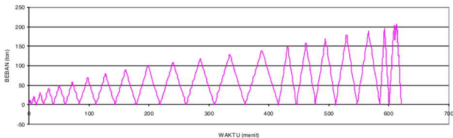
Gambar 4. Hubungan beban yang diberikan dan waktu pembebanan
