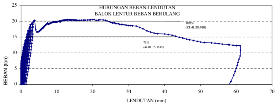
Gambar 5. Lup histerisis beban – lendutan
