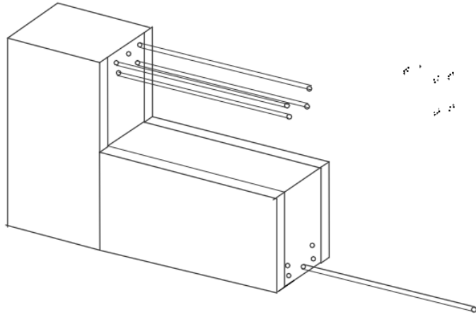
Gambar 1. Geometri sambungan takik
