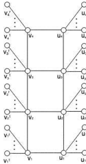
Gambar 1. Notasi Simpul Graf L_4 \odot \bar{K}_r
