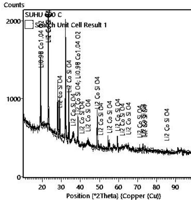
Gambar 2. Hasil identifikasi struktur kristal \text{Li}_2\text{CoSiO}_4 yang disinter pada suhu 600\text{ }^\circ\text{C} menggunakan program x'pert highscore plus .
