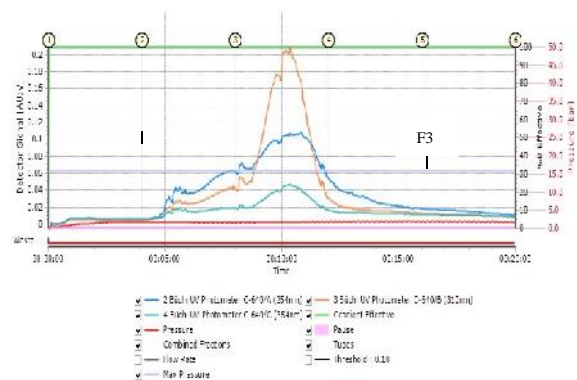
Gambar 4. Kromatogram MPLC ekstrak kasar air serbuk daun gamal KLU
