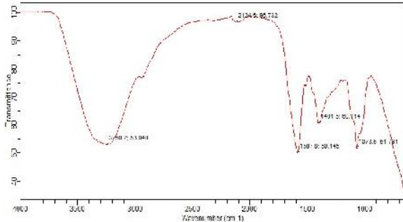
Gambar 10. Spektrum inframerah hasil isolasi
