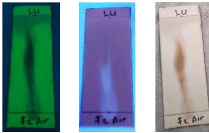
(a) (b) (c) Gambar 5. Kromatogram KLT dari fraksi 2 hasil MPLC ekstrak air serbuk daun gamal KLU (a) 254 nm AlCl 3 (b) 366 nm AlCl 3 (c) CeSO 4
