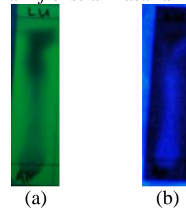
Gambar 3. Kromatogram KLT ekstrak kasar air serbuk daun gamal KLU pada panjang gelombang (a) 254 nm (b) 366 nm
