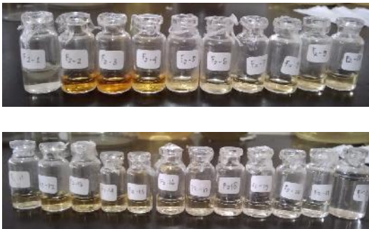
Gambar 6. Fraksi yang diperoleh dari kromatografi kolom C-18
