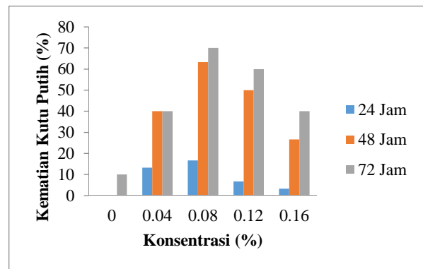
Gambar 11. Persentase kematian hama kutu putih ( P. minor ) pada buah kakao dengan perlakuan ekstrak kasar air serbuk daun gamal KLU pada konsentrasi dan waktu yang berbeda
