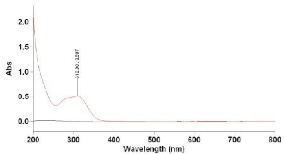
Gambar 9. Spektrum UV senyawa hasil isolasi
