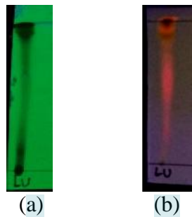
Gambar 1. Kromatogram KLT ekstrak kasar metanol serbuk daun gamal KLU pada panjang gelombang (a) 254 nm (b) 366 nm
