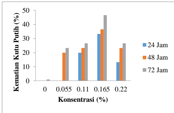
Gambar 12. Persentase kematian hama kutu putih ( P. minor ) pada buah kakao dengan perlakuan ekstrak murni air serbuk daun gamal KLU pada konsentrasi dan waktu yang berbeda
