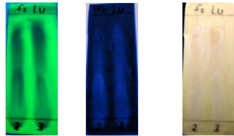
(a) (b) (c) Gambar 8. Kromatogram KLT fraksi 2 dan 3 kromatografi kolom (a) 254 nm AlCl 3 (b) 366 nm AlCl 3 (c) CeSO 4
