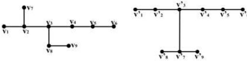
Gambar 4. Graf 3-etil-2-metil Heksana dengan 3-isopropil Heksana yang saling isomorfik
