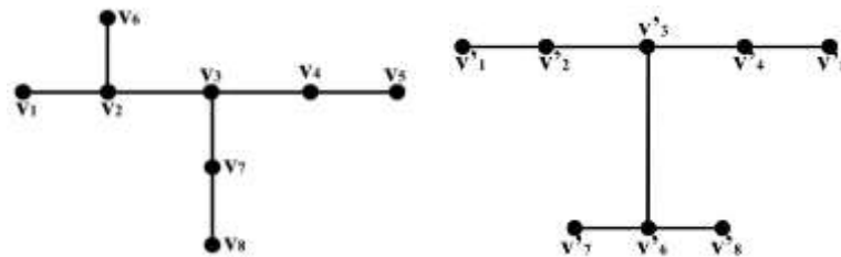
Gambar 3. Graf 3-etil-2-metil Pentana dengan 3-isopropil Pentana yang saling isomorfik
