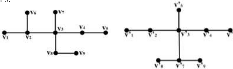
Gambar 5. Graf 3-etil-2,3-dimetil Pentana dengan 3-isopropil-3-metil Pentana yang saling isomorfik
