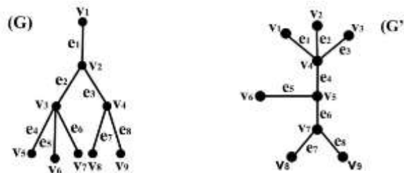
Gambar 1. Contoh Graf Isomorfik
