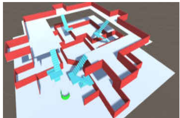
Gambar 10. Visualisasi 3D
