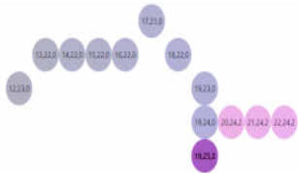
Gambar 9. Visualisasi Pathfinding
