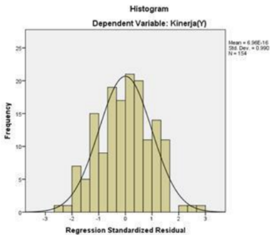
Gambar 1 Grafik Histogram
