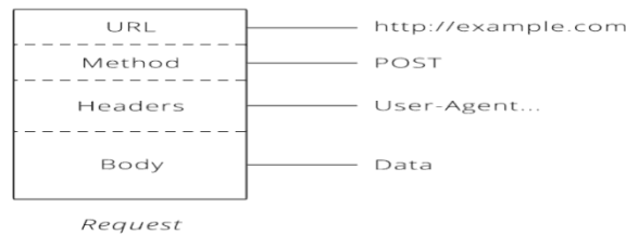
Gambar 5. Struktur HTTP Request
