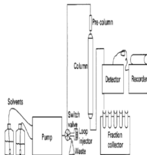
Gambar 2. Bagian alat MPLC
