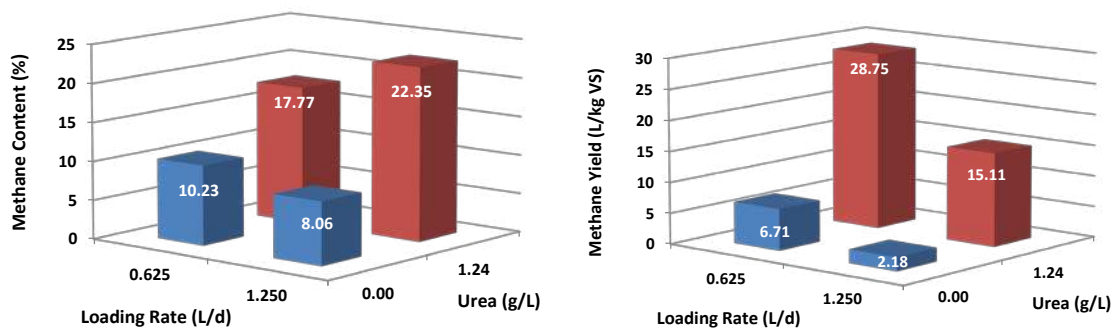
Gambar 10. Kandungan metana pada biogas dari campuran kotoran sapi dan rumput gajah dengan digester semi kontinyu.
