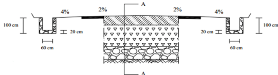
Gambar 4. Penampang melintang
