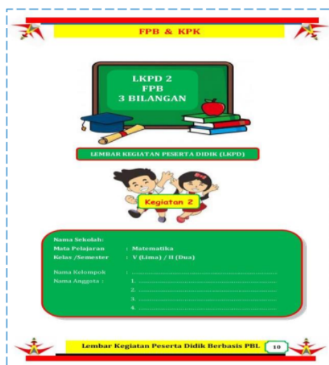
Gambar 1. Tampilan LKPD
