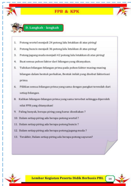
Gambar 3. Tampilan langkah-langkah
